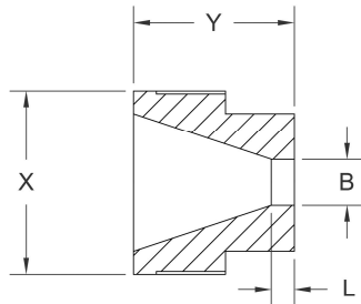
"B" STYLE ( NO DIE CUP)
